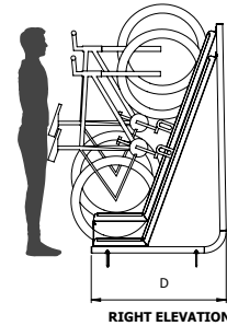
RIGHT ELEVATION
