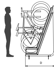
RIGHT ELEVATION
